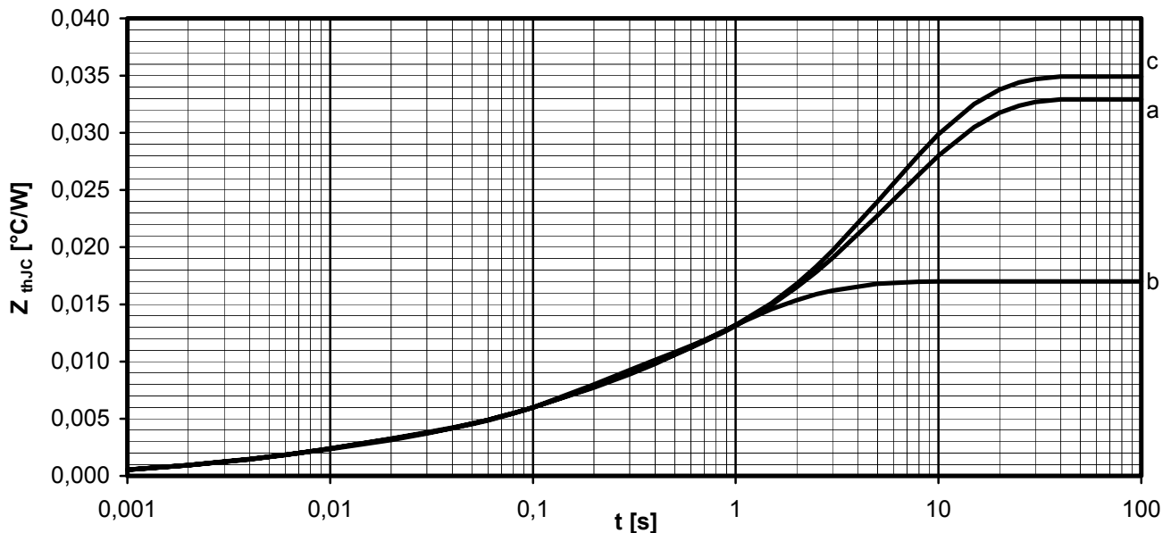
Transient innerer Wärmewiderstand für DC / Transient thermal impedance for DC Z_{thJC} = f(t)
